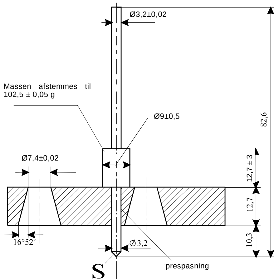
Fig. 4: Penetrometer
